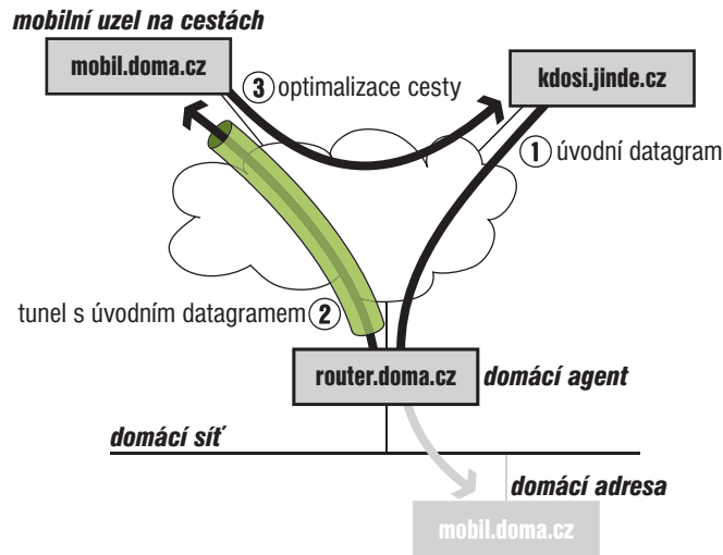
Obrázek 11.1: Navázání spojení s mobilním uzlem
