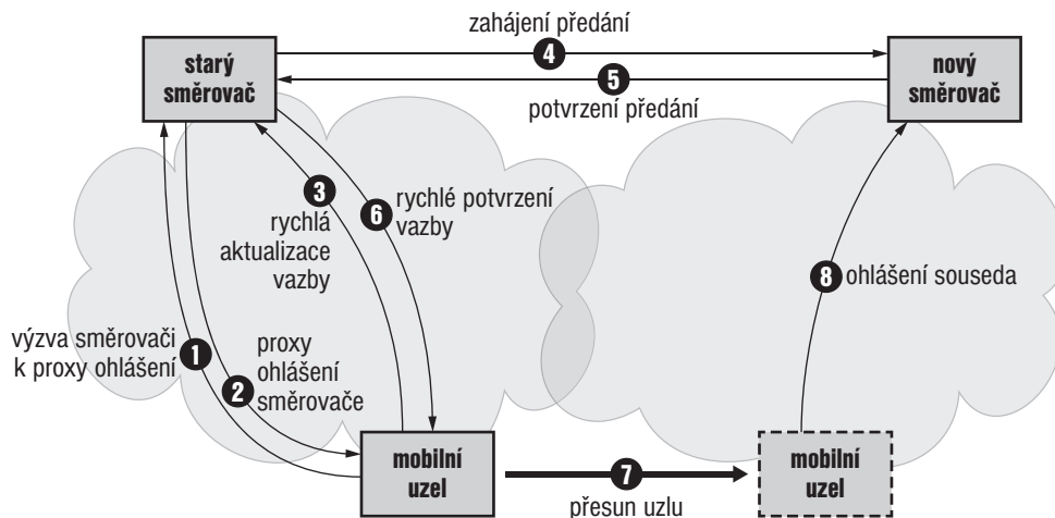
Obrázek 11.18: Rychlé předání
