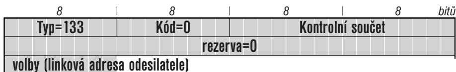
Obrázek 6.4: Výzva směrovači
