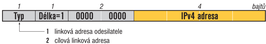
Obrázek 12.7: Volba Linková adresa pro objevování sousedů při 6over4
