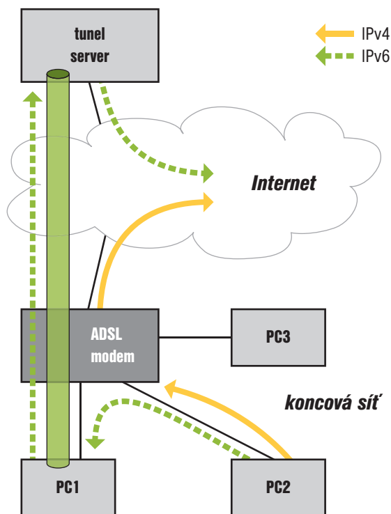
Obrázek 13.4: Nekonzistence směrování IPv4 a IPv6
