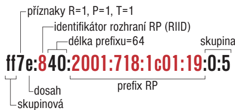
Obrázek 3.13: Příklad skupinové adresy obsahující RP
