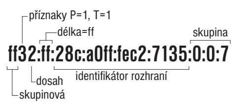
Obrázek 3.11: Příklad adresy založené na identifikátoru rozhraní
