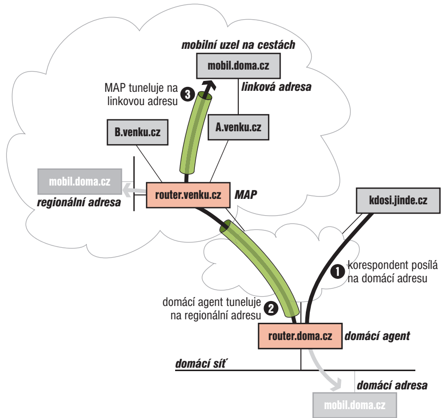
Obrázek 11.19: Hierarchická mobilita
