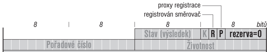
Obrázek 11.23: Rozšířené příznaky v Potvrzení vazby
