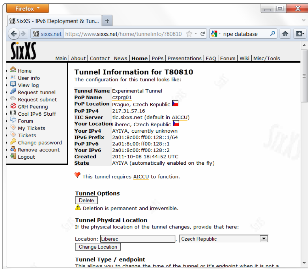
Obrázek 13.2: Parametry tunelu u SixXS
