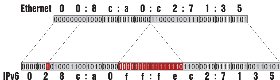
Obrázek 3.2: Vytvoření modifikovaného EUI-64 z ethernetové adresy
