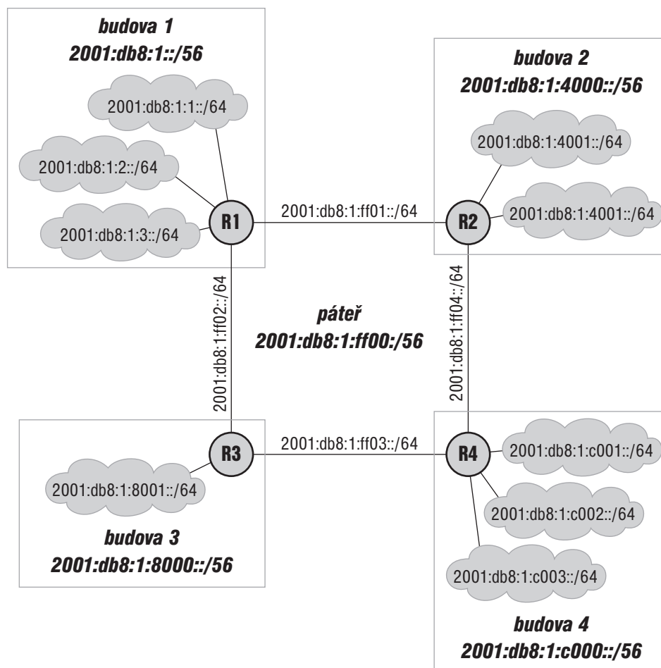
Obrázek 13.7: Příklad hierarchicky uspořádaných identifikátorů podsítí
