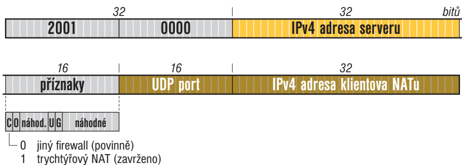
Obrázek 12.9: Struktura adresy pro Teredo
