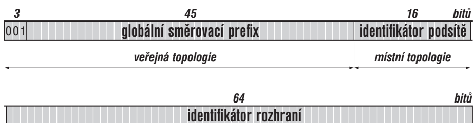
Obrázek 3.1: Obvyklá struktura globální individuální adresy
