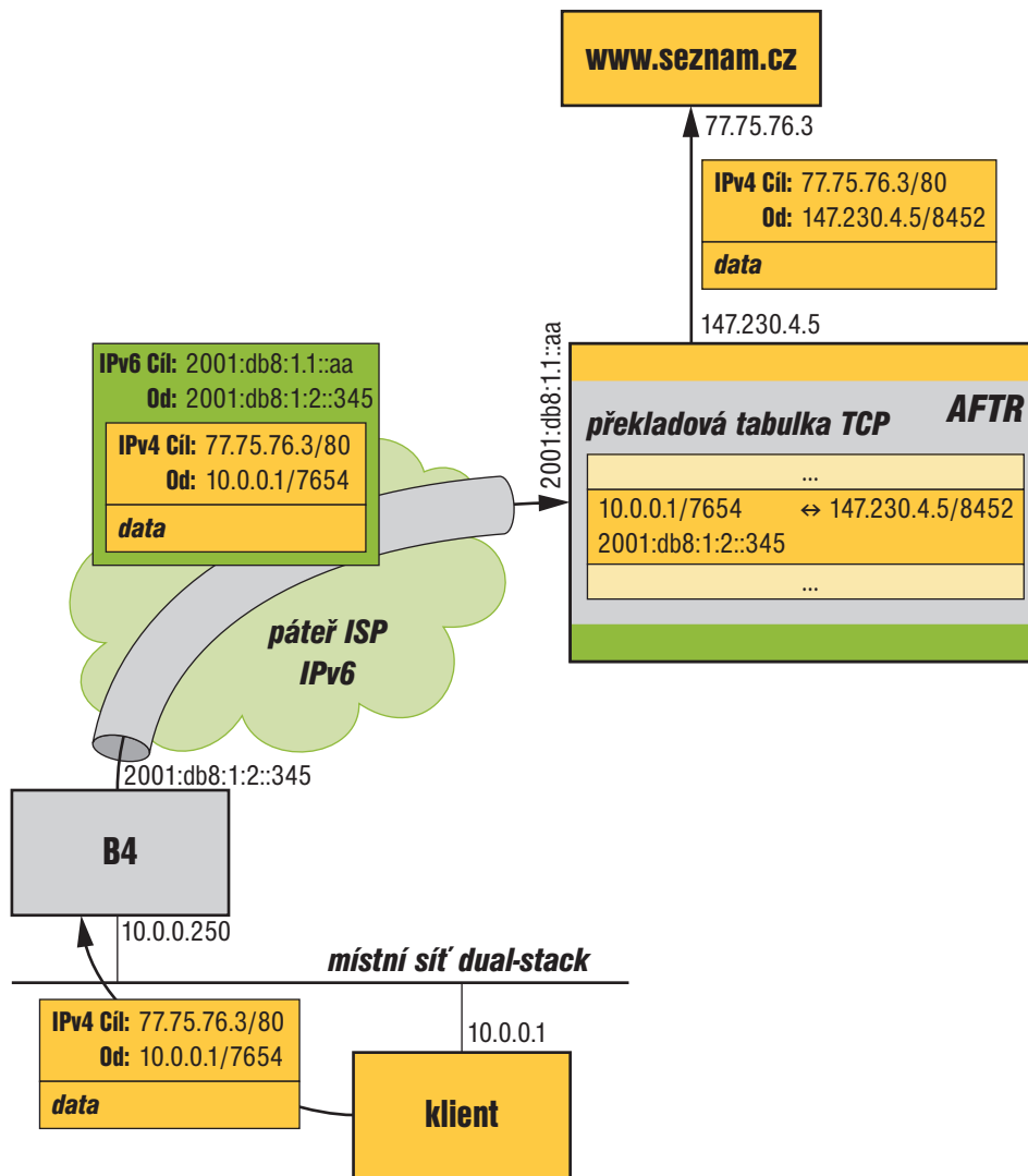
Obrázek 12.11: Dual-stack lite
